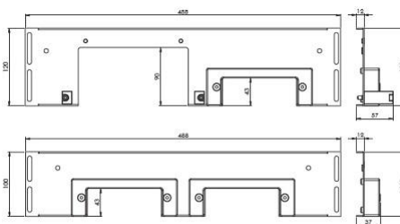
KDR-ESR-VX25 für Rittal VX25
